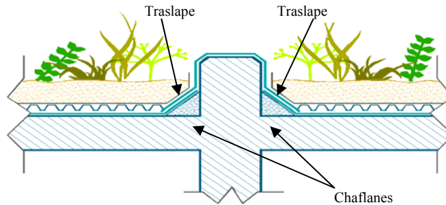
Figura 4. Impermeabilización en puntos de encuentro con elementos emergentes intermedios por debajo del nivel del sustrato o de altura menor a 10cm sobre el nivel del mismo.
