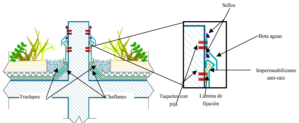
Figura 2. Impermeabilización con membrana prefabricada asfáltica en puntos de encuentro con elementos emergentes intermedios. (Los sellos deberán ser de materiales impermeables como el silicón o poliuretano)
